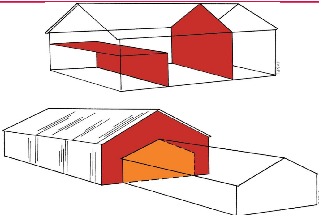
Figur 4.5a 3.5a Exempel på brandavskiljande konstruktioner brandcellsgränser.
