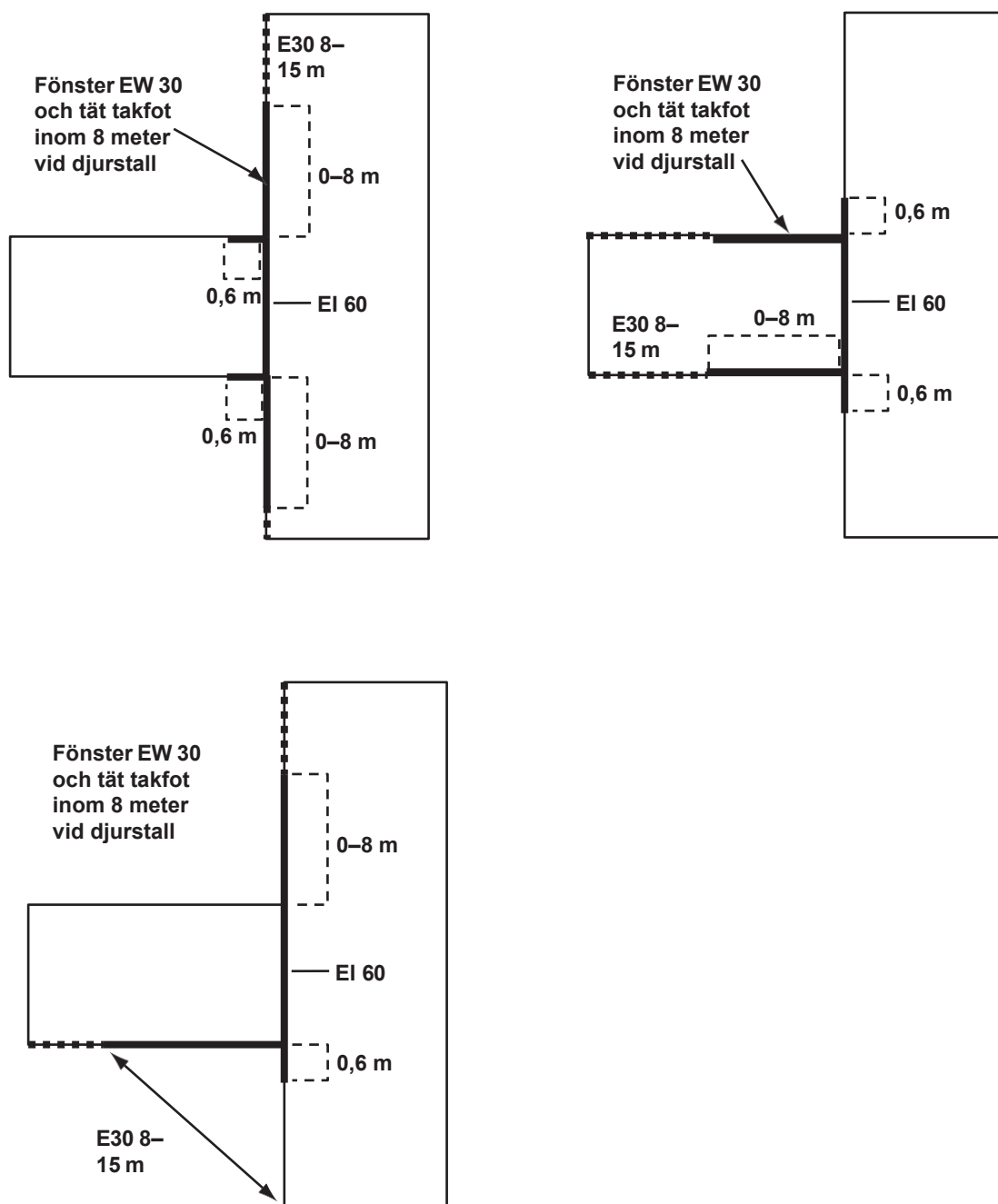
Figur 4.3c 3-3e Olika exempel på hur vinkelsmitta kan förhindras. Notering till förlaget & läsare. Figur 4.3c har ändrat utformning (ska vara två bilder bredvid varandra). Nedersta bilden tas bort.
