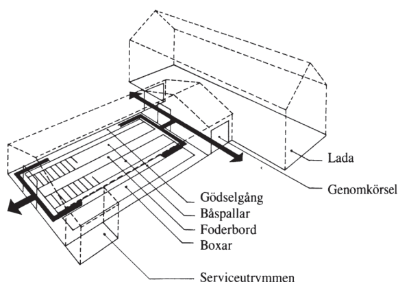
Figur 3.2a 2.2a Exempel på utrymningsvägar.
