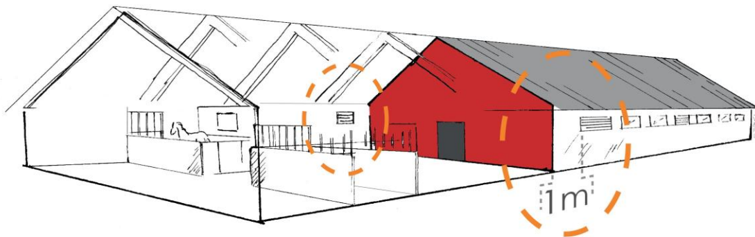
Figur 5.3.1.a 4.3.1.a Ventilationsöppning vid takfoten ska placeras minst en meter från brandavskiljning brandcellsgräns.
