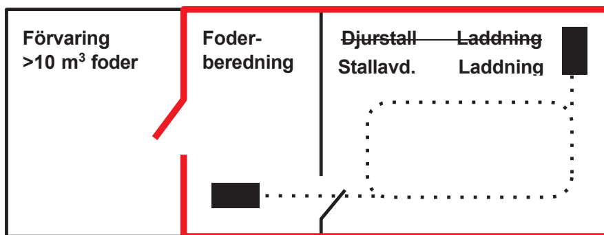
Figur 6.1.5 c 5.1.5 c Exempel på fodervagn i utrymme för foderberedning i avskilt utrymme men inom samma brandcell som stallavdelningen djurstallet . I foderberedningsutrymmet får det förvaras högst 10 m 3 foder och strö.
