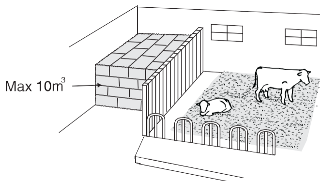
Figur 6.1.6 c 5.1.6 c Avbalkat mellanlager i stallavdelning djurstall får rymma högst 10\text{ m}^3 .
