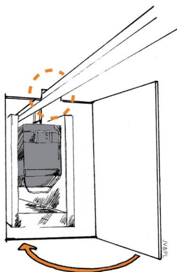
Figur 6.1.5 a 5.1.5 a. Exempel på fodervagnsräls som passerar vägg som inte är brandklassad. Med särskild tätning godtas även lösningen för brandklassad vägg.
