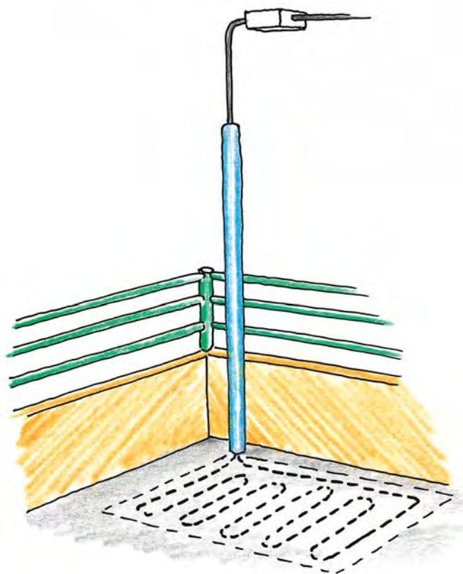
Bild 15. Anslutningsledningar till golvärmeinstallationer måste skyddas med till exempel OMG-rör där det finns risk att djuren kan skada dem.
