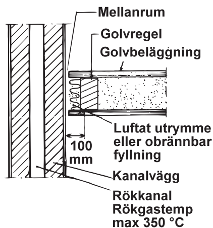
Fig 5.2 Bjälklagsanslutning till röckkanal
