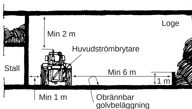
Fig 2.4 Uppställning av dieselmotordrivna fordon i maskinhall och loge.
