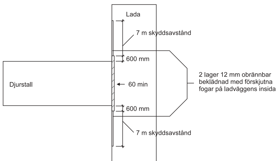
Figur Bil 2.6 Detalj av anslutning mellan djurstallsvägg i trä och ladvägg i plåt.
