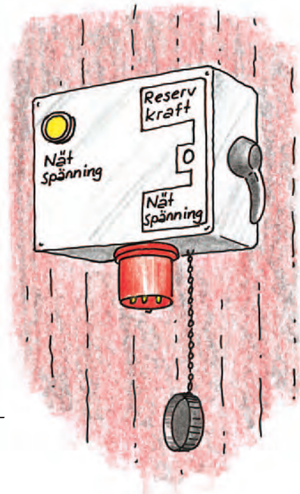
Bild 31. Mobila reservverk ansluts vanligtvis via speciella reservkrafttag. Även om man inte har ett eget reservverk rekommenderas att man installerar reservkrafttag i samband med nybyggnad eller större ombyggnad av elinstallationen.
