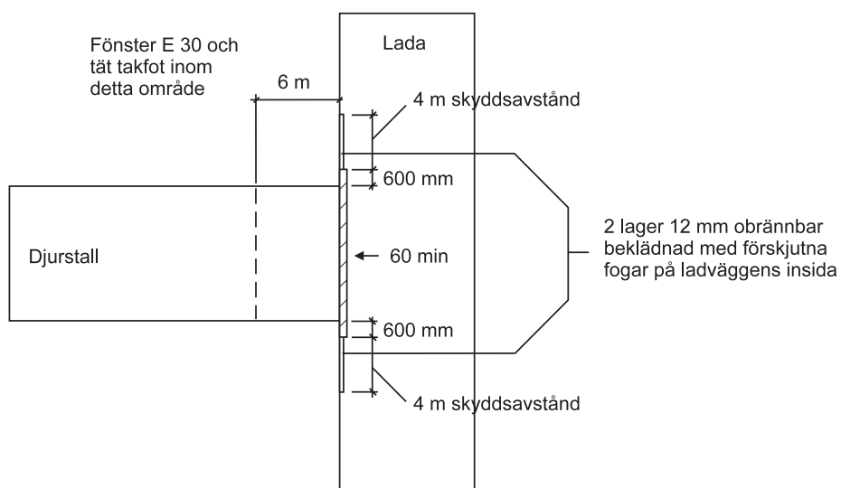
Figur Bil 2.5 Detalj av anslutning mellan djurstallsvägg i plåt och ladvägg i plåt.
