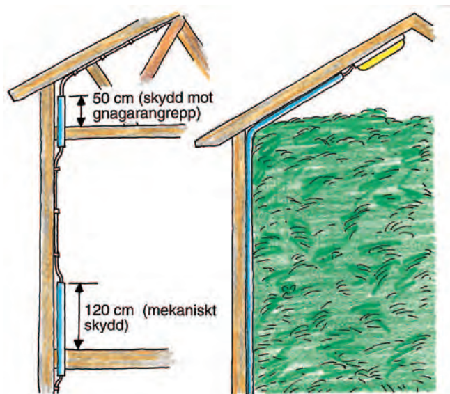
Bild 6. Vid genomgångar i bjälklag i utrymmen där det finns risk för råttangrepp ska kablarna skyddas minst 50 cm över den horisontella ytan. Mekaniska skydd bör sträcka sig minst 120 cm över golvet.
