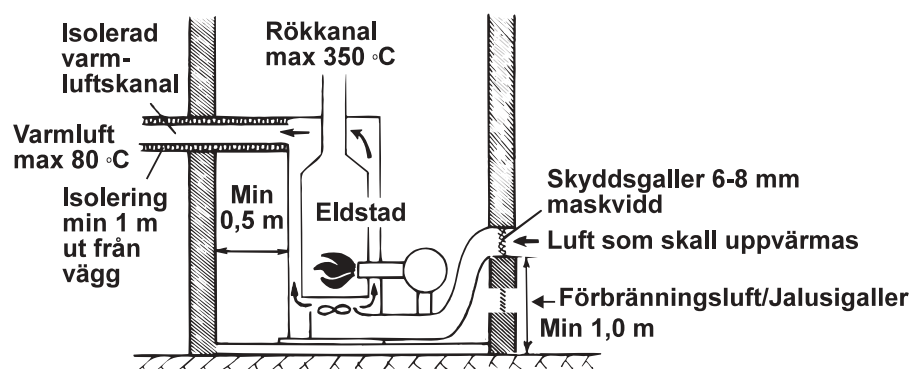
Fig 3.6 Principskiss för installation av värmepanna
