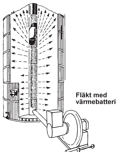
Fig 9.3.3 a Av LBK godkänd elvärmefläkt använd som ensam värme- och luftkälla till en silotork
