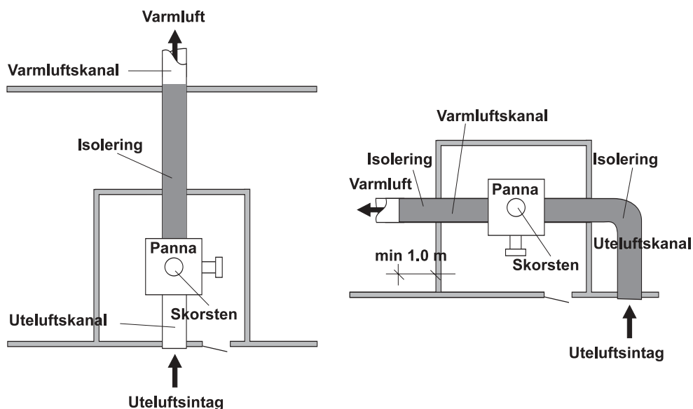
Fig 6.3.2 och Fig 6.3.3. Planskiss pannrum m m.
