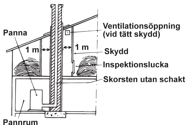
Fig. 4.1 Särskilt skydd kring rökkanal
