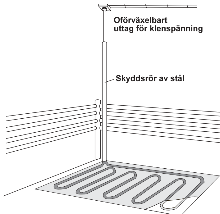
Fig 8.8 Värmebädd
