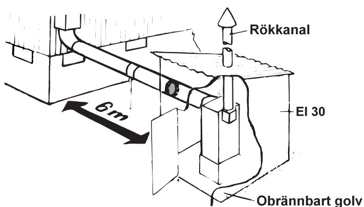
Fig 2.1.2 Fristående pannhus
