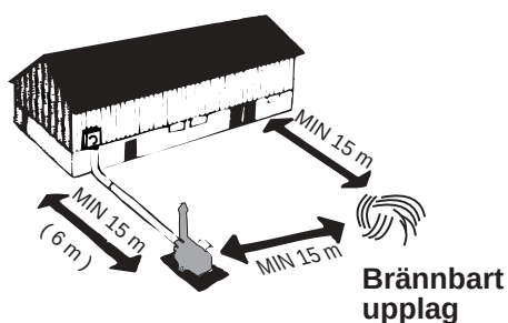
Fig 2.1.3 Värmepanna under bar himmel
