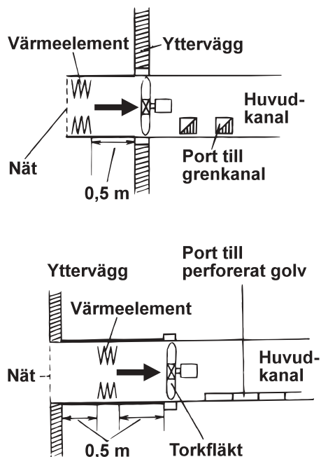
Fig 9.3.1 b Elvärmebatteri (högst 20 kW) utan egen fläkt utanför vägg
