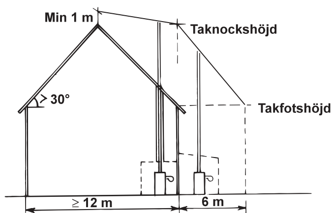
Fig 4.6.2 b Reducering av rökkanals höjd inom 6 m breda byggnader med branta tak.
