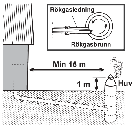
Fig 4.8.3 Rökgasbrunn
