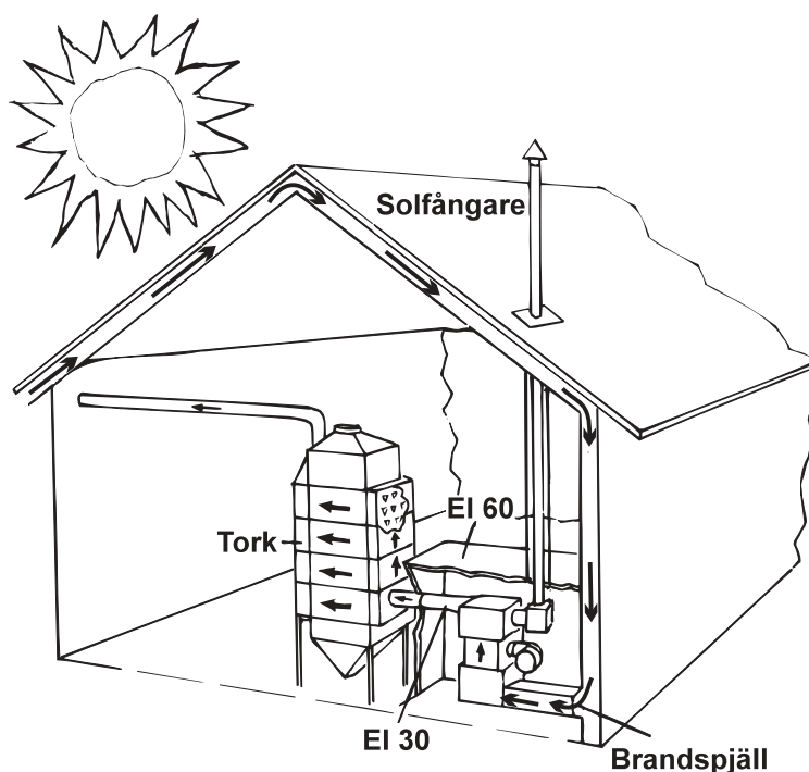
Fig 9.1 Principskiss av varmluftstork med solfångaruppvärmd tilluft
