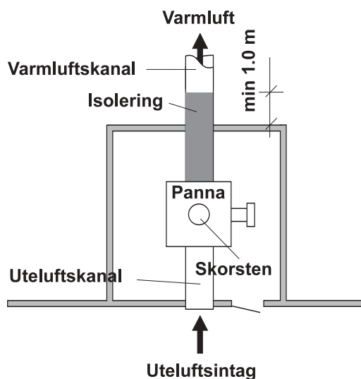
Fig 6.3.1. Planskiss pannrum m m.
