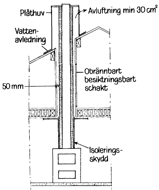
Figur 4.5.1 Lätt schakt
