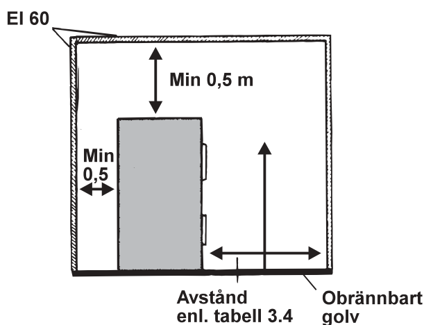
Fig 2.1.4 Uppställning av värmepanna (gäller även fastbränslebehållare)
