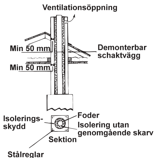
Fig 4.3.1 Rökkanal isolerad i hela sin längd
