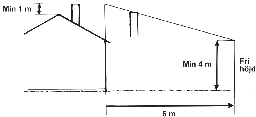
Fig 5.3 Avgaskanals höjd
