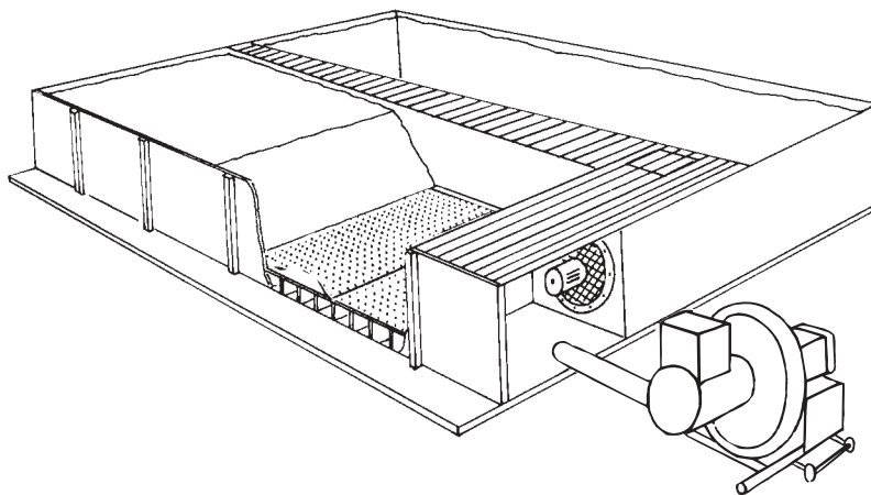
Fig 9.3.3 b Av LBK godkänd elvärmefläkt använd som tillsatsvärmekälla till en plantork.
