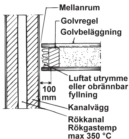
Fig 4.2 Bjälklagsanslutning till röckanal
