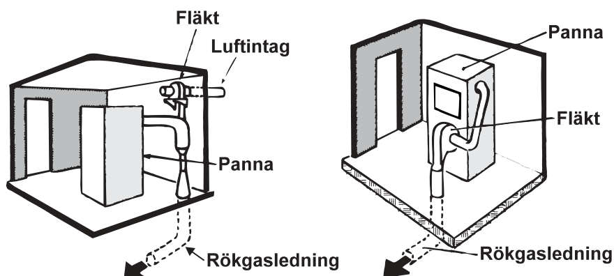
Fig 4.8.1 Rökgasledning och rökgasfläkt med respektive utan injektor.
