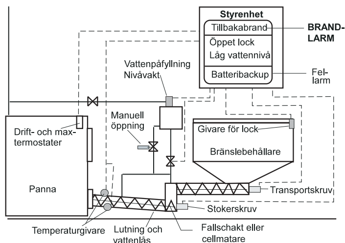
Fig 2.1.5 Exempel på skydd vid automatisk fastbränsleledning
