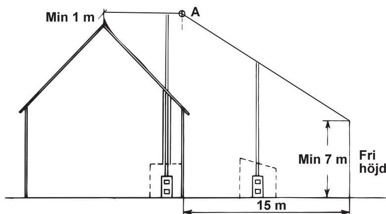
Fig 4.6.3 Rökkanals höjd vid fastbränsleeldning
