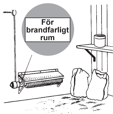
Fig 8.4 Elkamin med övertäckningsskydd
