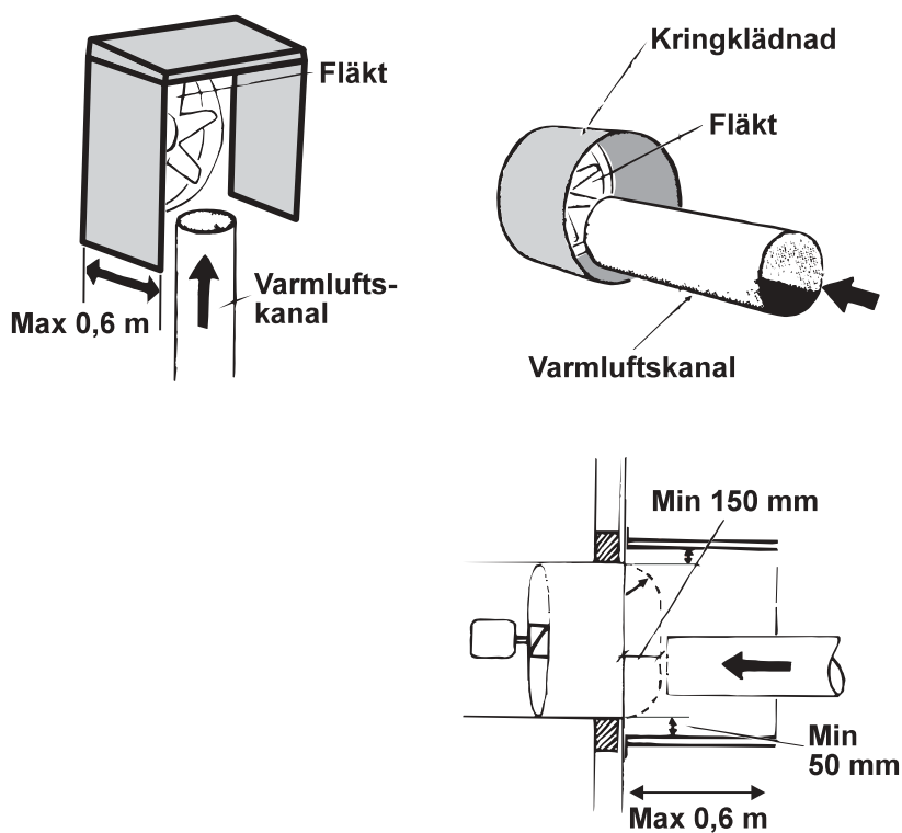
Fig 3.6.1 a-c Dragavbrott
