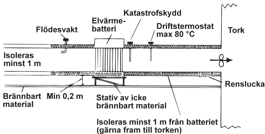
Fig 9.3.1 a Principskiss för driftskydd vid elvärmeanläggning över 20 kW till tork
