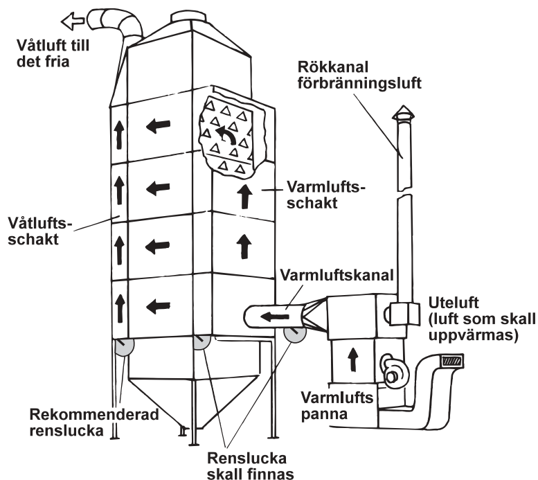
Fig 9.2 Principskiss för varmluftstork
