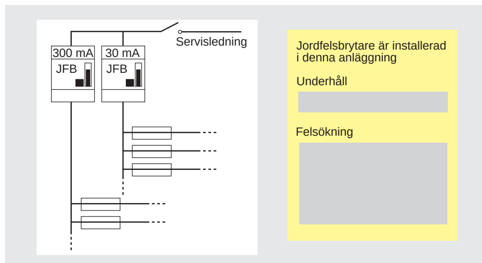
Bild 22. Vid jordfelsbrytarna bör det finnas anvisningar om hur ofta brytarna ska provas, hur man gör vid eventuella fel samt ett schema över vilka grupper respektive jordfelsbrytare skyddar.
