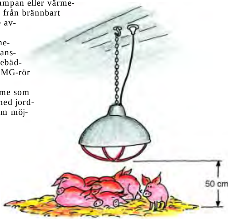
Bild 14. Uttagen för värmelampor och värmetak ska monteras så att stickproppen dras ur om värmaren faller ned. Lampan ska hänga minst 50 cm från brännbart material om inte tillverkaren föreskriver annat.
