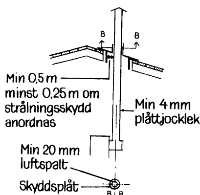
Fig 4.3.2 Oisolerad rökkanal genom yttertak
