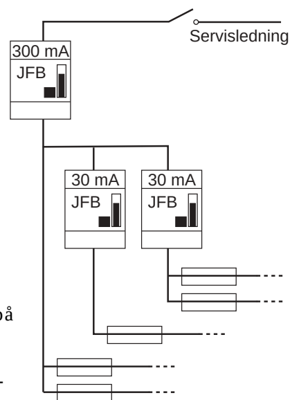
Bild 21. Om jordfelsbrytarna kopplas i serie måste den överliggande vara en så kallad selektiv jordfelsbrytare med tidsfördröjd utlösning.
