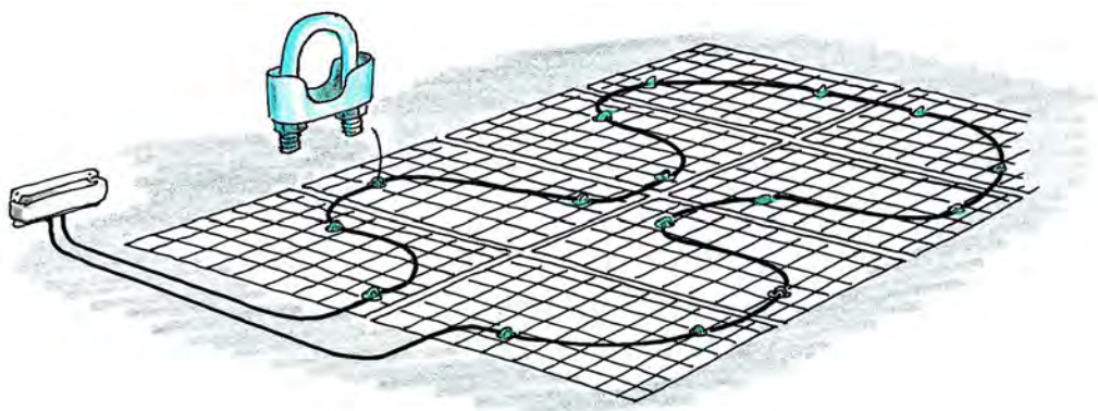
Bild 26. Potentialutjämningsledarna till armeringen i golvet bör läggas i slinga och fästas med vajerlås för att få god elektrisk förbindelse.
