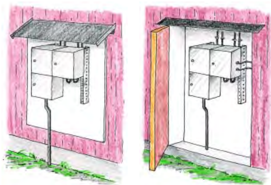
Bild 16. Centraler bör i första hand placeras i separata elrum, i torra och dammfria utrymmen eller i nischer, alternativt på så sätt att de inte utsätts för direkt solljus och regn. Där det finns risk för kondensproblem bör de monteras på distans, 5 till 10 cm.
