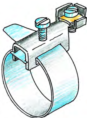
Bild 27. Potentialutjämningsledarna kan anslutas till inredningen med hjälp av speciella anslutningband.
