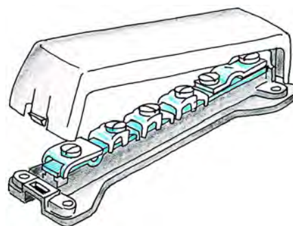
Bild 25. Potentialutjämningsledarna bör kopplas samman på en separat huvudjordningsskena.
