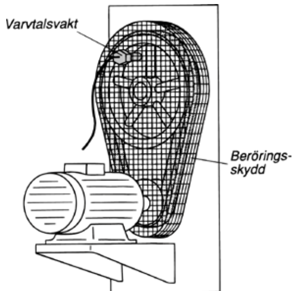
Remtransmission med varvtalsvakt och beröringskydd.
