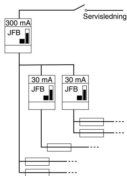
Figur 18a. Om jordfelsbrytare kopplas i serie bör den överliggande vara en så kallad selektiv jordfelsbrytare med tidsfördröjt frångslag för att minska driftstörningar.
