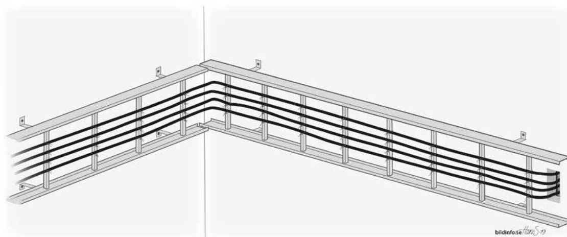
Horisontal stega vertikalt monterad. Kablar ska vara najsade.
