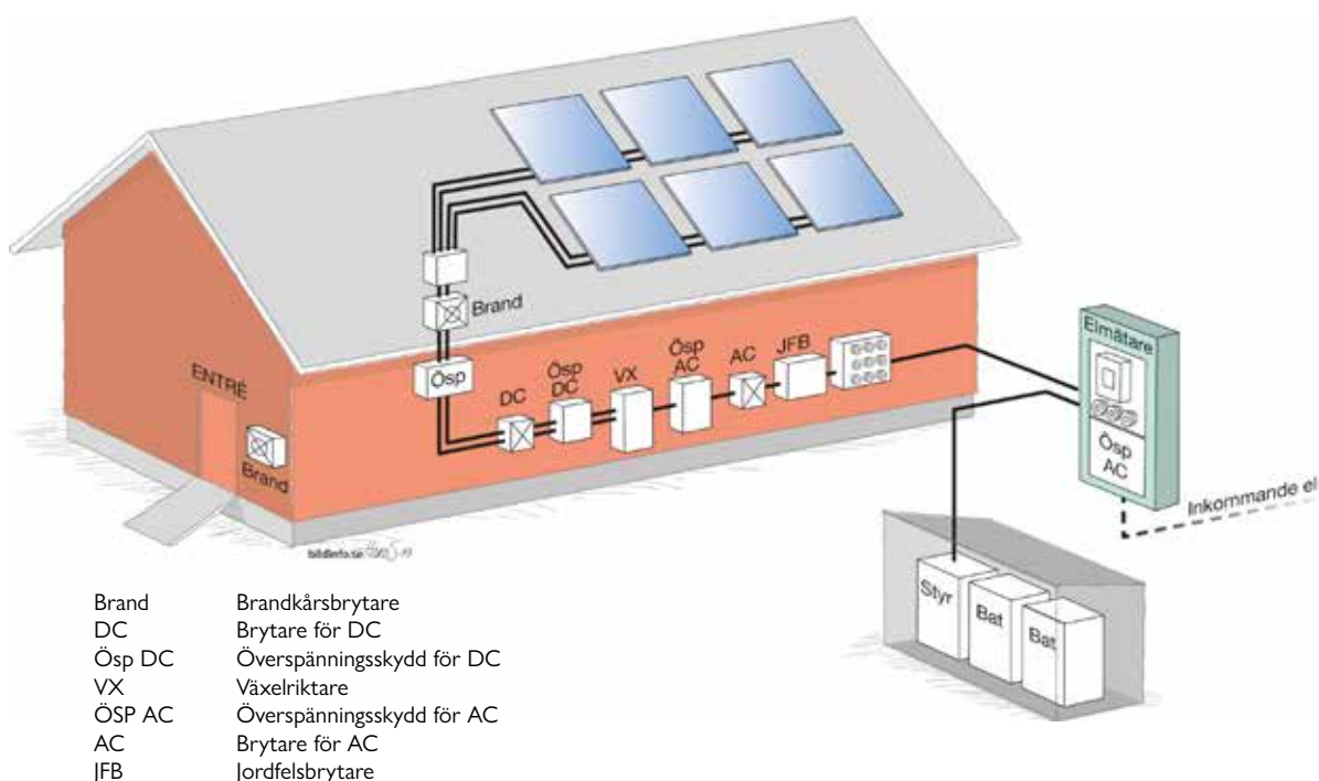
Figur 24a. Principskissen visar vilka funktioner som krävs på en större anläggning. Vissa funktioner kan anordnas gemensamt.
