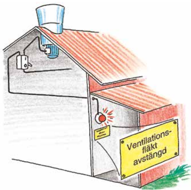
Figur 13. Där funktionen är mycket viktig bör det finnas indikering om att lastfrånkopplaren är frånslagen.
