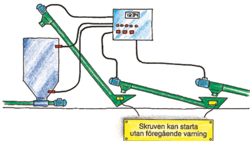
Figur 14. Utrustning som fjärrstyrs eller startas automatiskt måste försees med varningsskyltar.
