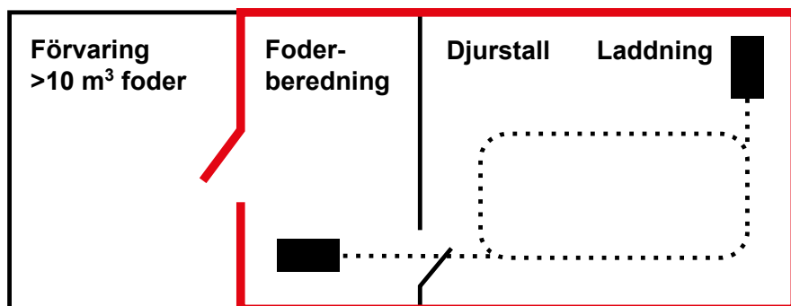
Figur 5.1.5 c Exempel på fodervagn i utrymme för foderberedning i avskilt utrymme men inom samma brandcell som djurstallet. I foderberedningsutrymmet får det förvaras högst 10 m³ foder och strö.
