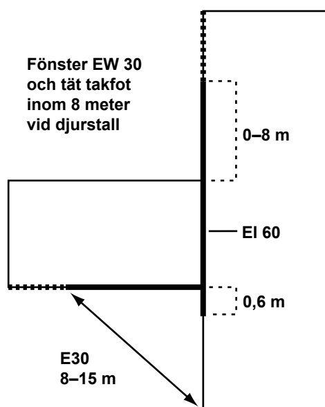
Figur 3.3c Olika exempel på hur vinkelsmitta kan förhindras.
