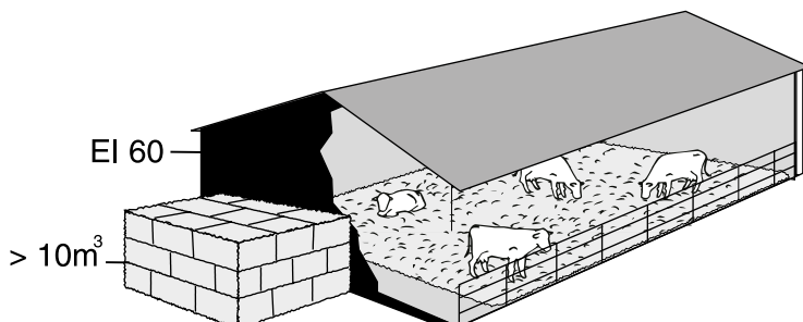
Figur 5.1.6 a Om lager överstiger 10\text{ m}^3 ska väggen utföras i lägst brandteknisk klass EI 60.
