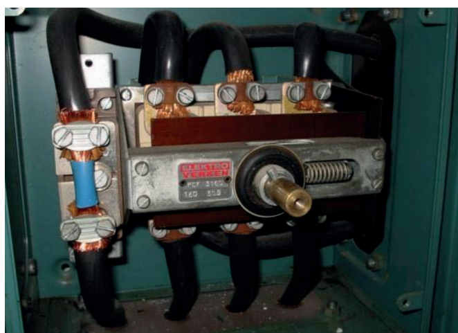
På bilden passerar PEN-ledare genom en delbar nollplint. Plinten har efter en anmärkning vid revisionsbesiktning förbikopplats.
