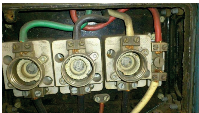
På bilden passerar PEN-ledare genom en delbar nollplint
