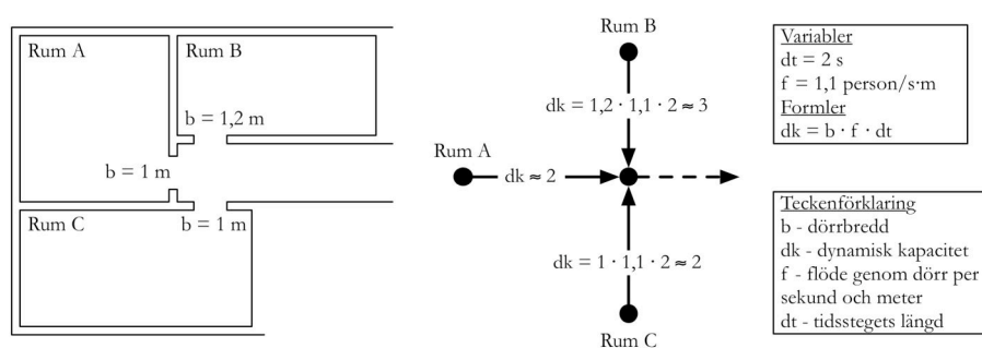
Figur 3. En bit av en byggnad och motsvarande nätverk i EVACNET4. Den dynamiska kapaciteten ( dk ) för kopplingarna har beräknats utifrån flödet för dörren ( f ), dörrbredden ( b ) och tidsstegets längd ( dt )
