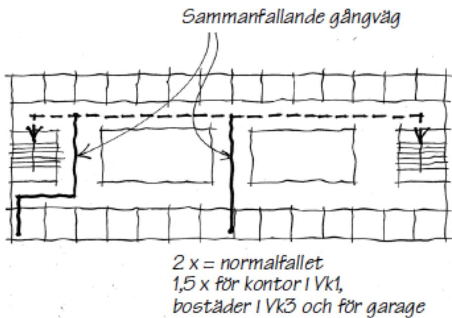
Figur 9: beräkning av gångavstånd (hämtad från Brandskyddshandboken med tillåtelse).
