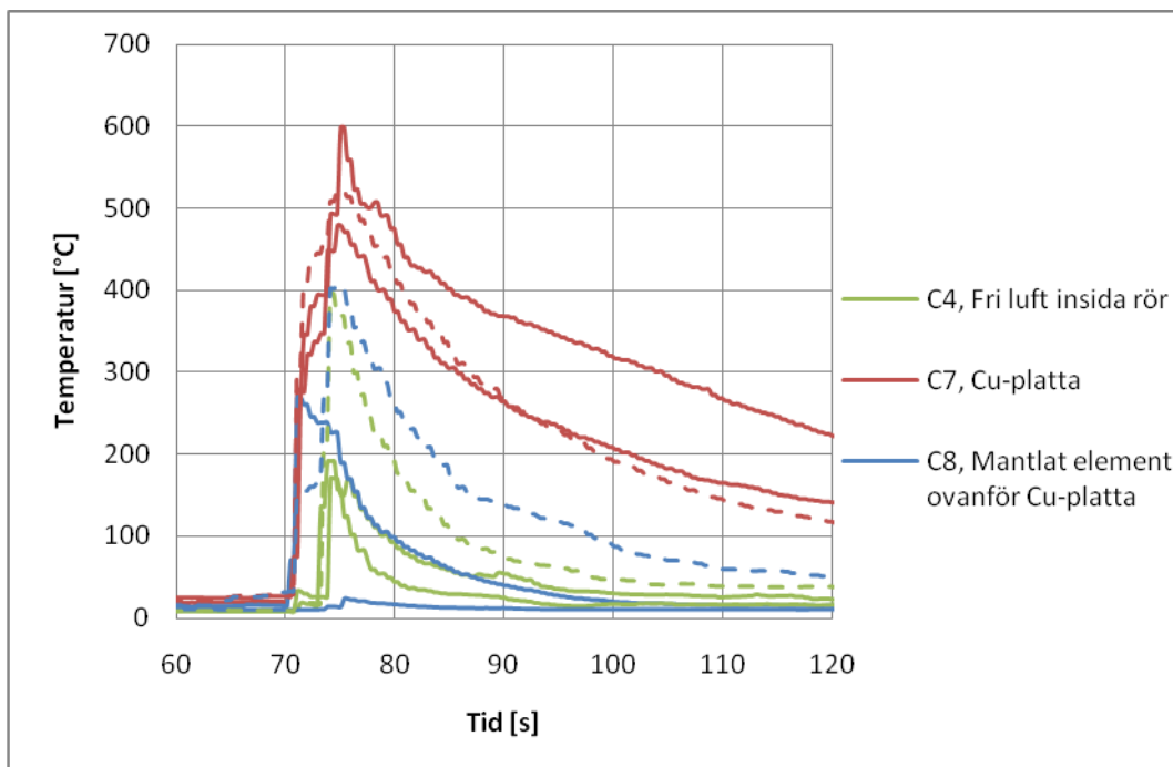
Figur 21 Variation mellan test 6-7 och test 10, d.v.s. fyrverkeripjäsen MegaTwin. Försöken med kortare styrpinne (17 cm jämfört med 22 cm) visas med streckad linje.
