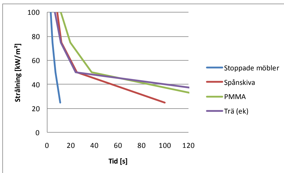
Figur 26 Tid till antändning för olika strålningsnivåer i konkalorimetern
