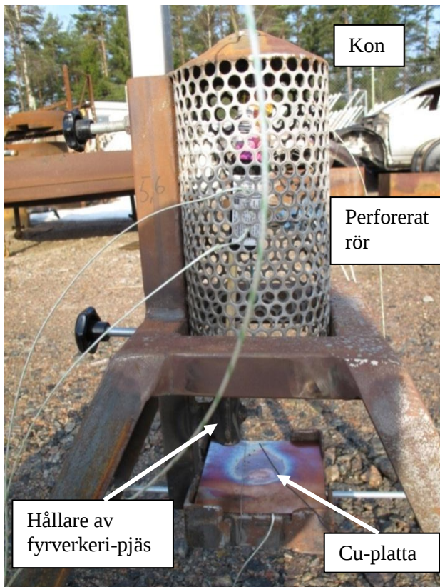
Figur 5 Testrigg
